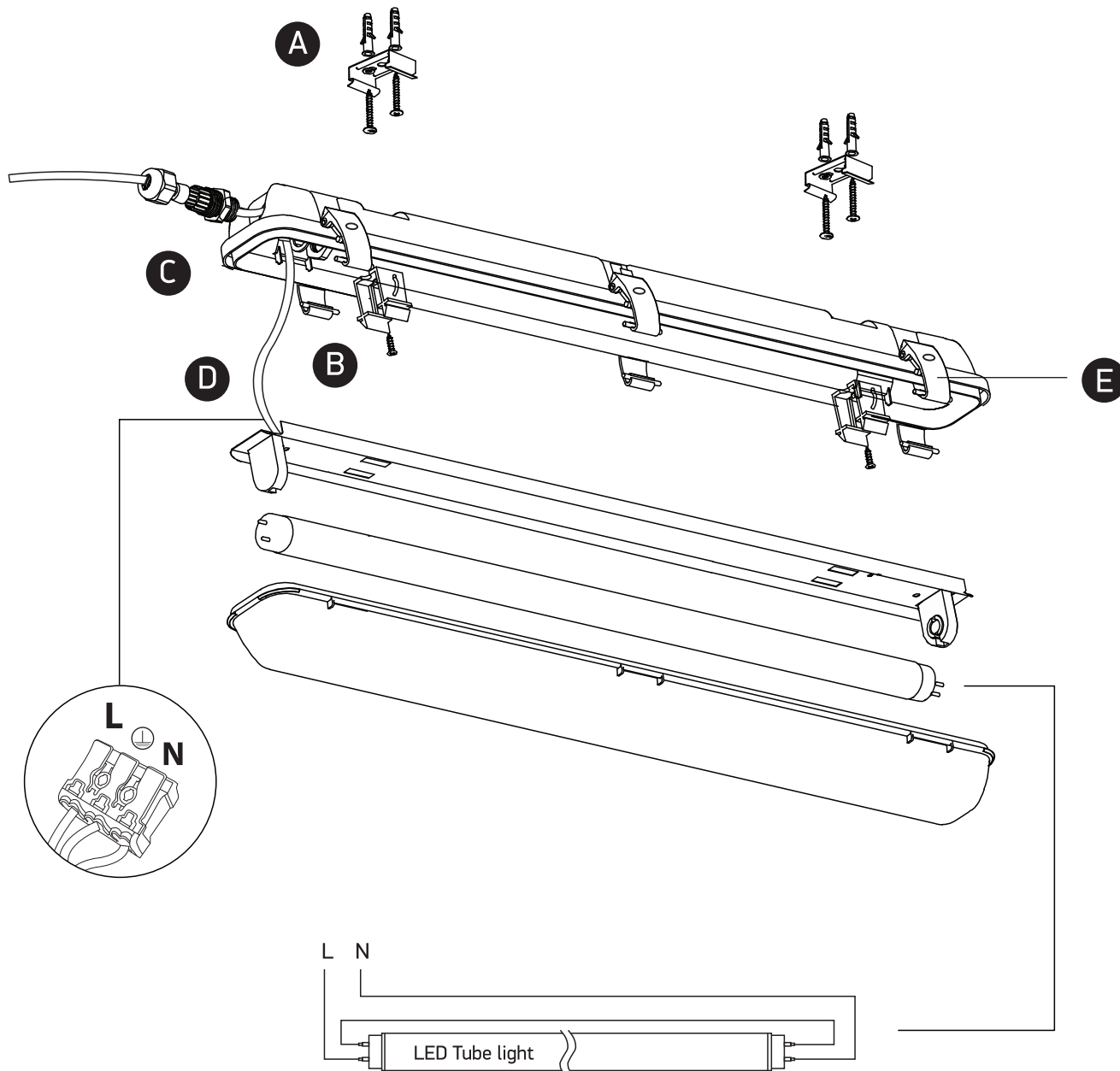
Wiring diagram.
