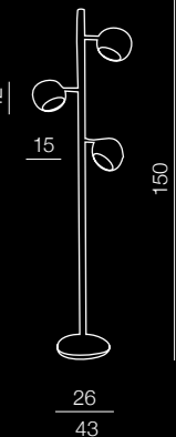
Trinton AZ0024 E14 3x 40W metal chrome
