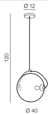
Rufus 40
